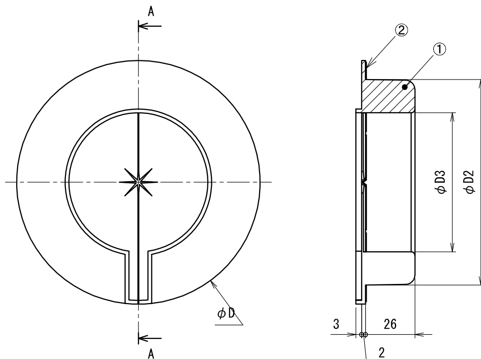
断面A-A
